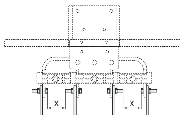
Образец крепления болтов
