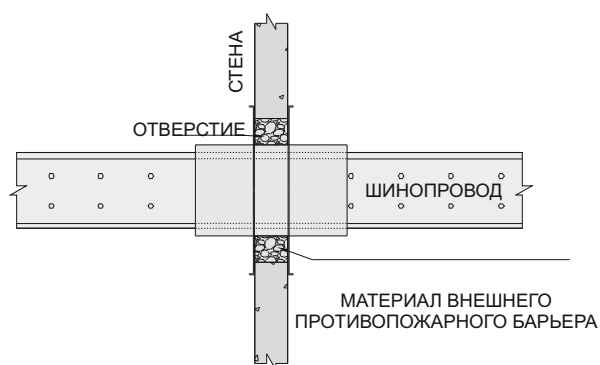
РИСУНОК-5 ПРИМЕР ПЕРЕСЕЧЕНИЯ СТЕНЫ С ПРОТИВОПОЖАРНЫМ БАРЬЕРОМ
