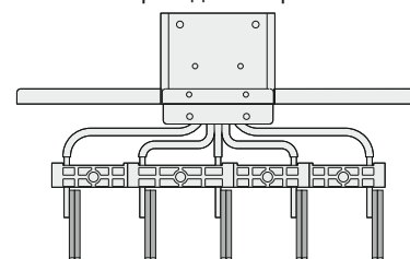
Образец крепления проводников фаз
