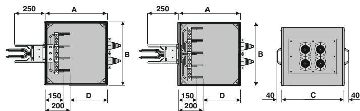
двух- и трехсторонняя система, 4 проводника
