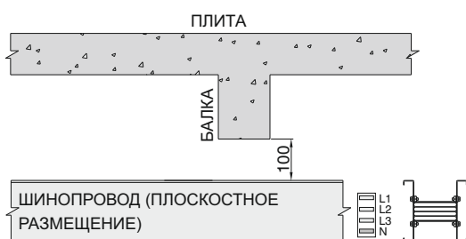
РИСУНОК-4 ПЕРЕСЕЧЕНИЕ ПОД БАЛКОЙ А В ГОРИЗОНТАЛЬНОМ РАЗМЕЩЕНИИ
