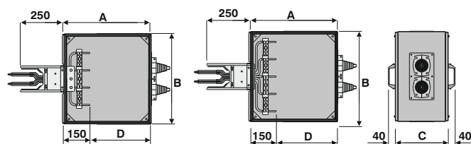
Односторонняя система, 4 проводника
