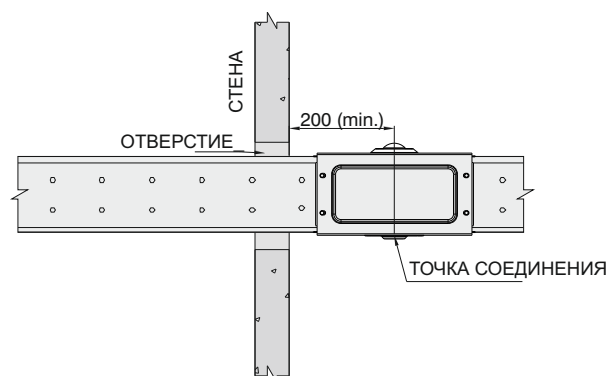
РИСУНОК-6 ПЕРЕСЕЧЕНИЕ СТАНДАРТНОЙ СТЕНЫ
