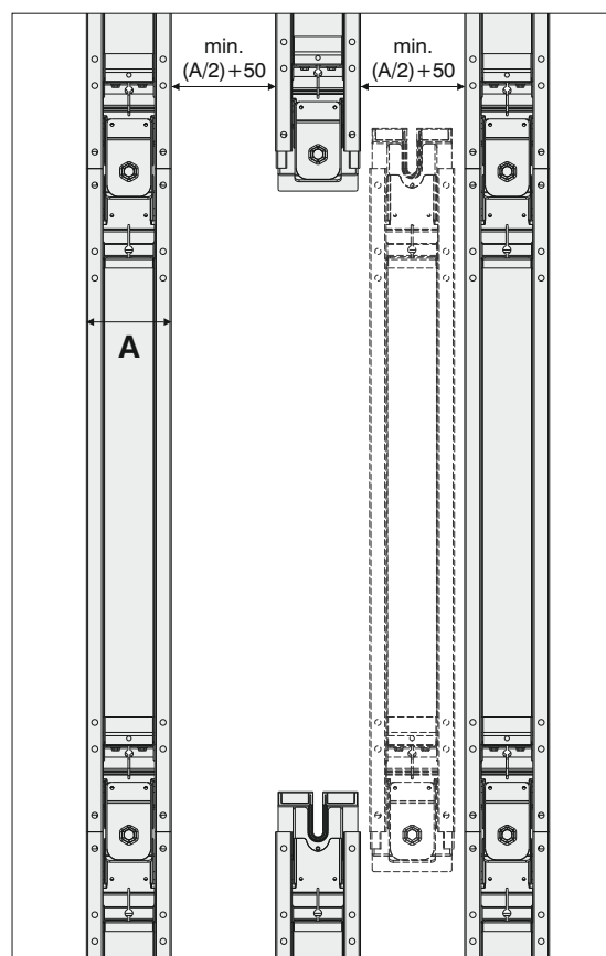
МИНИМАЛЬНОЕ РАСТОЯНИЕ МЕЖДУ ЛИНИЯМИ ШИНОПРОВОДА В ГОРИЗОНТАЛЬНОМ ПРИМЕНЕНИИ
