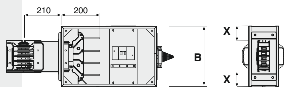
Ответственная коробка с компактным выключателем
